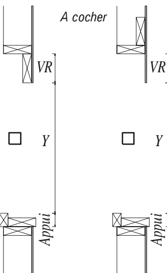
Coupe Verticale avec VR
