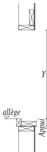
Coupe Verticale sans VR
